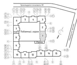
Схема блока/блочки
