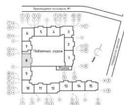
Схема планировки
